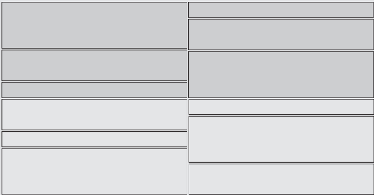
modulo module A | spazzolato 30x119,8 rt - 2 pz. 20x119,8 rt - 2 pz. 10x119,8 rt - 2 pz.
